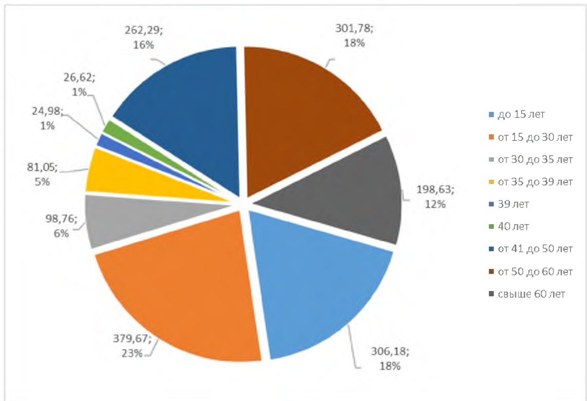
Рисунок 13 Протяженность и срок эксплуатации распределительных газопроводов
