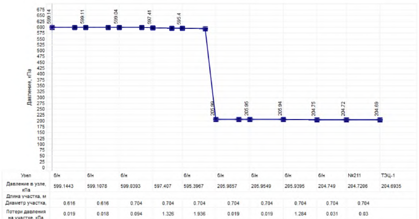
Рисунок 97 График падения давления от ГРП Тимашево до ТЭЦ-1
