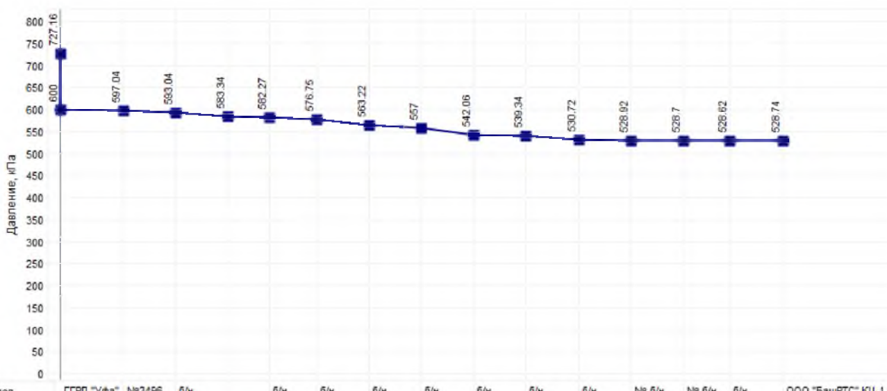
Рисунок 83 График падения давления от ГГРП Тимашево до ТЭЦ-1
