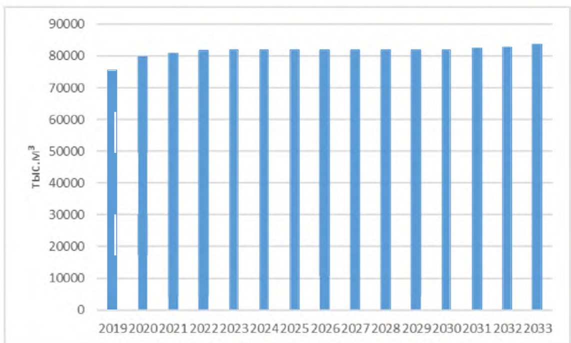
Рисунок 59 Расход газа по КЦ-3 на 2019-2033 гг.
