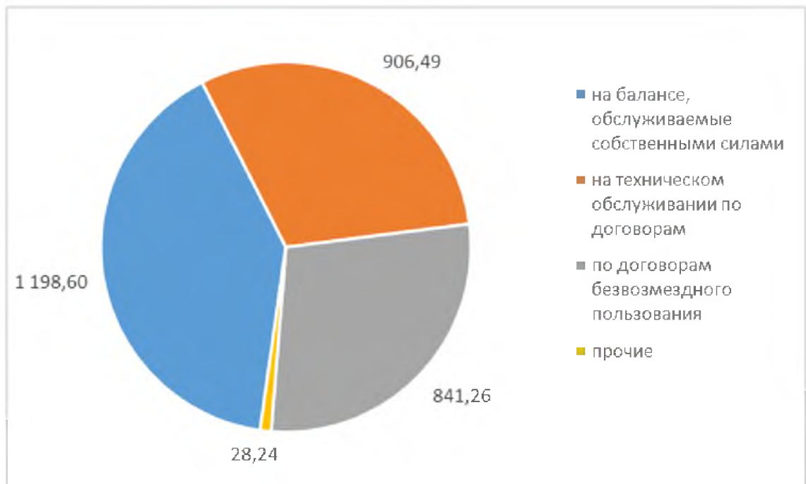
Рисунок 12 Протяженность наружных газопроводов по имущественной принадлежности, км
