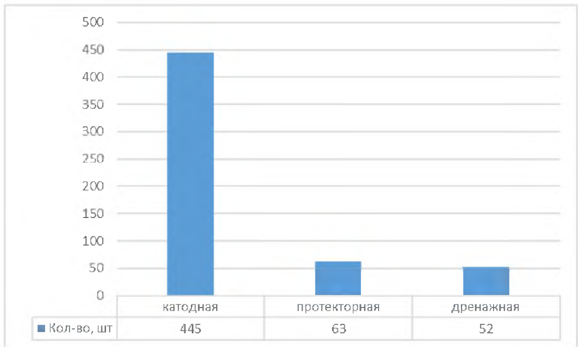
Рисунок 14 Характеристики установок электрохимической защиты
