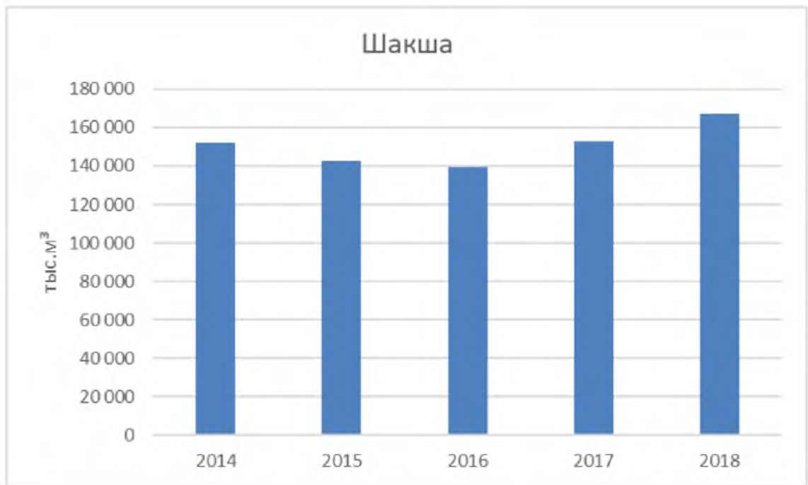
Рисунок 36 Фактическая производительность ГРС «Шакша» в 2014-2018 годах
