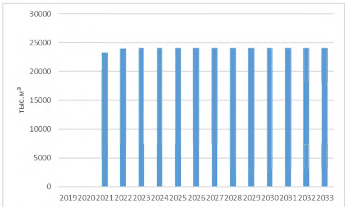
Рисунок 62 Расход газа по котельной «Глумилино» на 2019-2033 гг.
