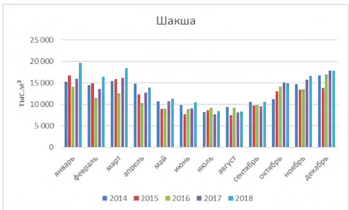
Рисунок 37 Помесячная производительность ГРС «Шакша» в 2014-2018 годах
