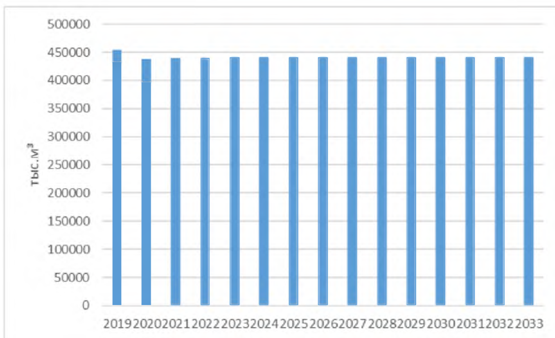
Рисунок 53 Расход газа по ТЭЦ-3 на 2019-2033 гг.
