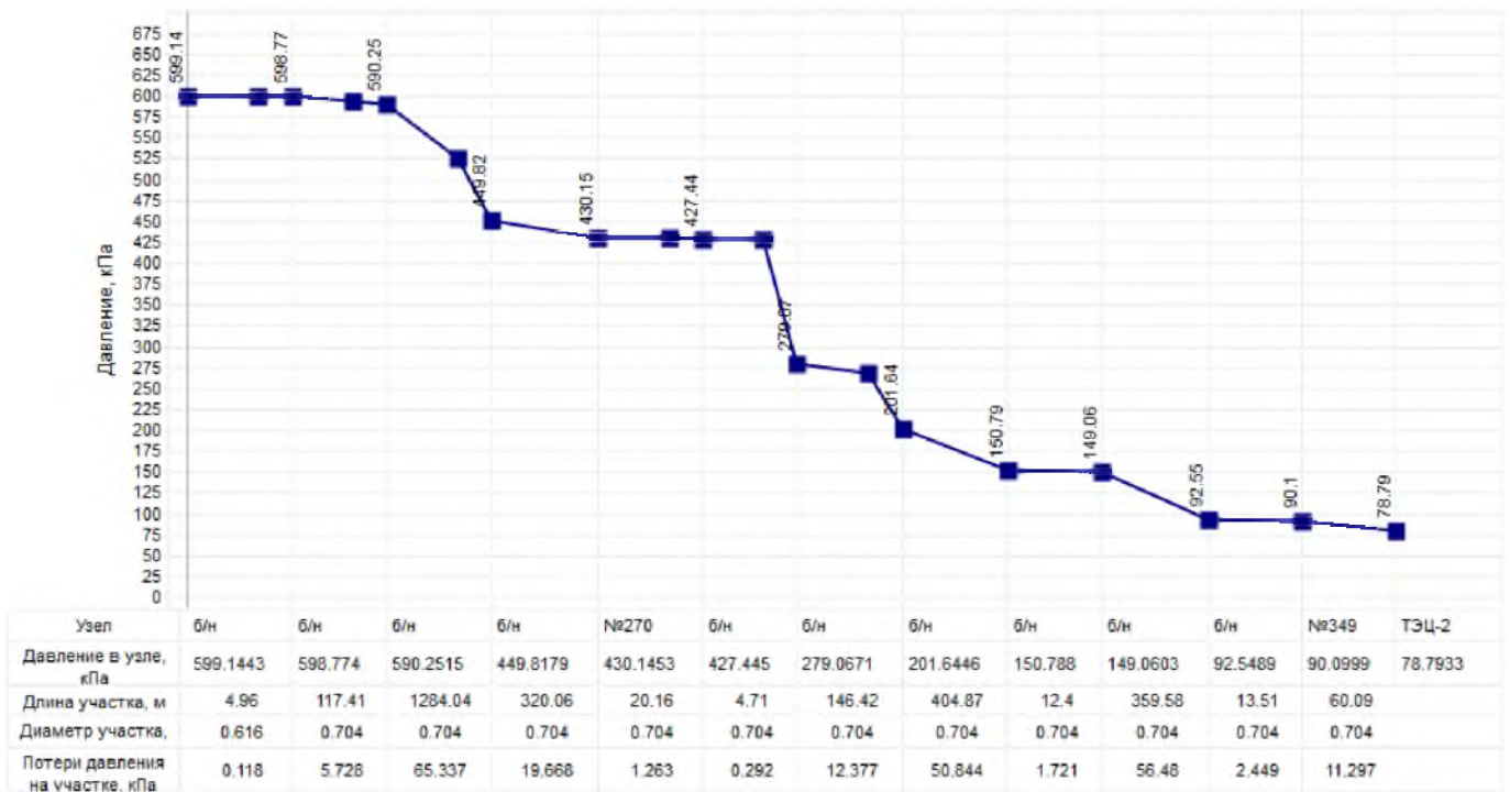
Рисунок 96 График падения давления от ГРП Тимашево до ТЭЦ-2
