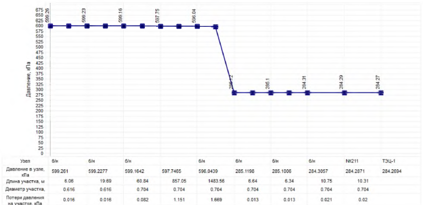
Рисунок 94 График падения давления от ГРП Тимашево до ТЭЦ-1
