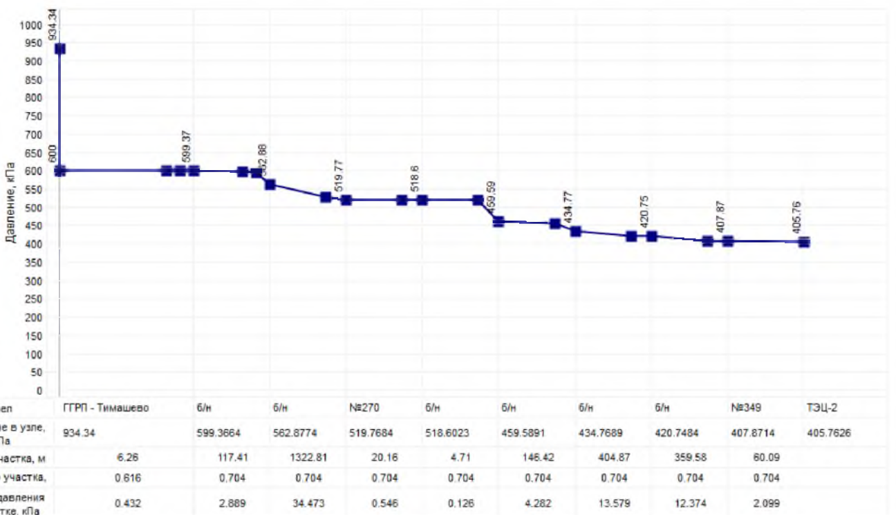
Рисунок 82 График падения давления от ГГРП Тимашево до ТЭЦ-2
