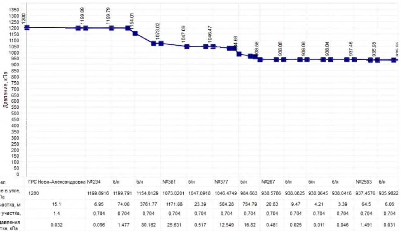
Рисунок 81 График падения давления от ГРС Ново-Александровка до ГГРП Тимашево
