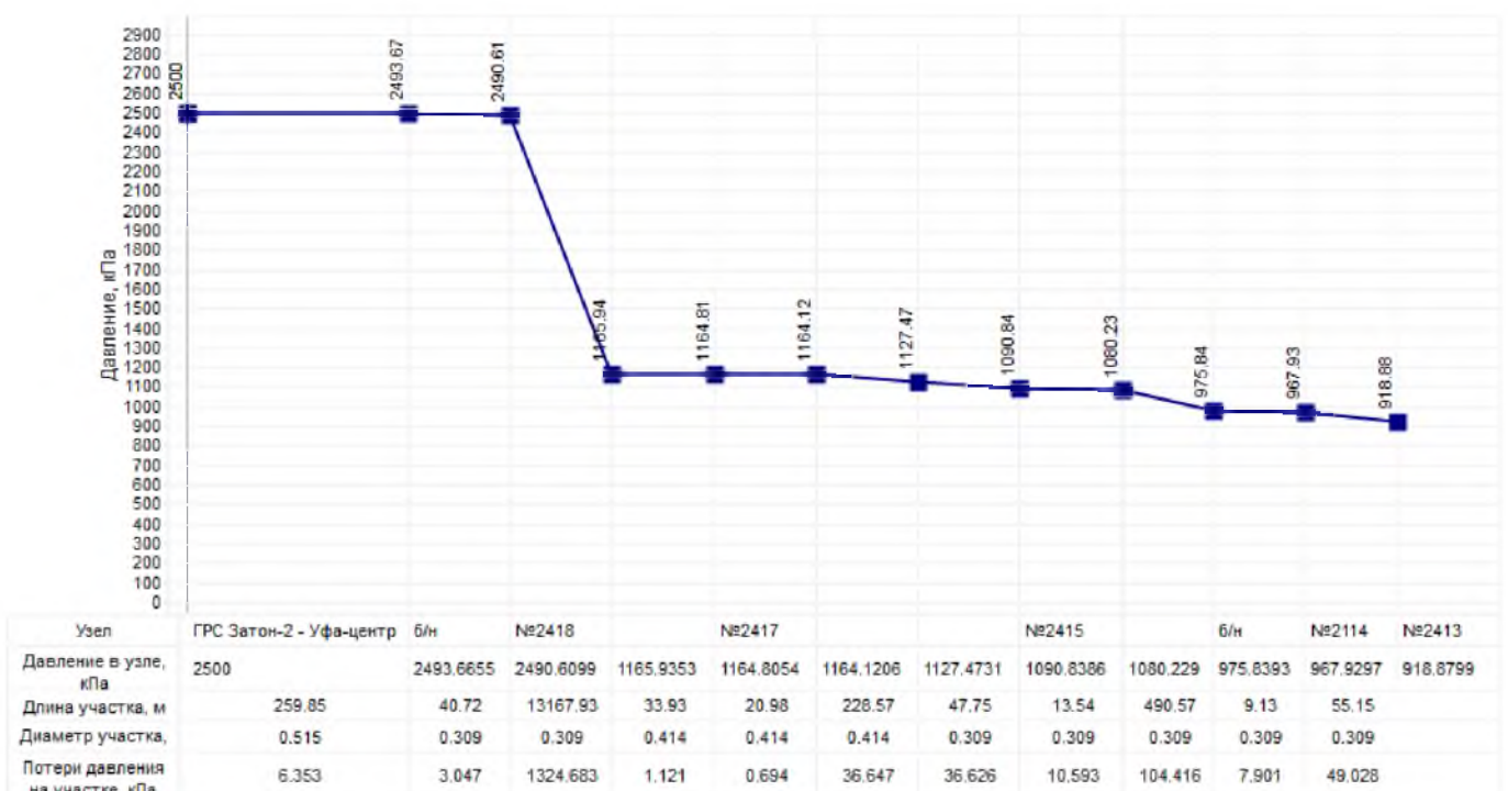
Рисунок 95 График падения давления от ГРС Затон-2 до ГРП Уфа
